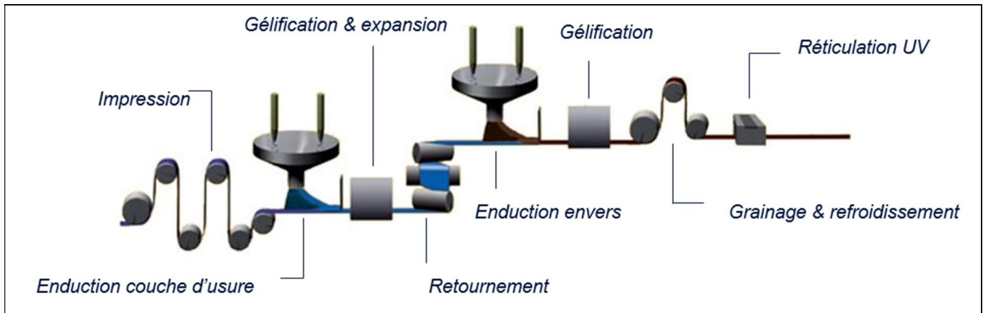
Figure 1 : Processus d'Enduction
